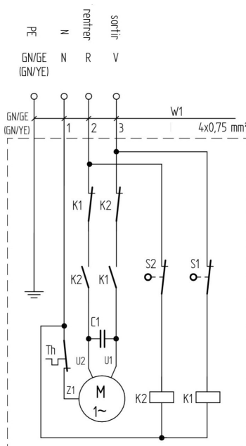
Protection thermique Fin de course «tige sortie» Fin de course «tige rentrée»
