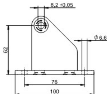
PALIER ARRIERE: 29031-1
