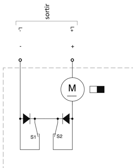
S1 Tige «sortie» S2 Tige «rentrée»
